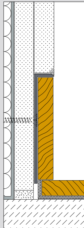
Unterschnittener Einbau (höhenversetztes Profil) mit Holz- / Laminatboden
