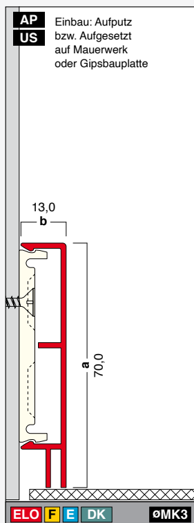
G70-13-DK Höhe: 70,0 mm Breite: 13,0 mm Länge: 4,0 m
