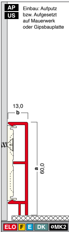
G60-13-DK Höhe: 60,0 mm Breite: 13,0 mm Länge: 4,0 m
