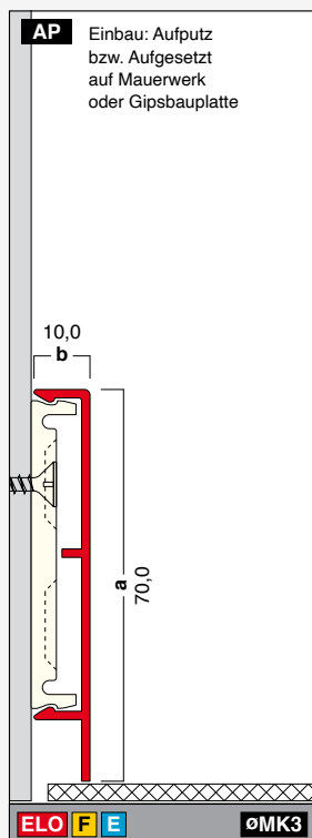
G70-10 Höhe: 70,0 mm Breite: 10,0 mm Länge: 4,0 m
