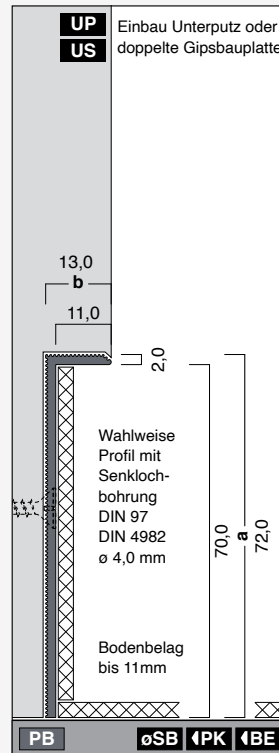
B72-13-BE11-RF-PB Höhe: 72,0 mm Breite: 13,0 mm Länge: 4,0 m
