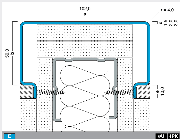
WA-E Edelstahl-Wandabschluss im Trockenbau
