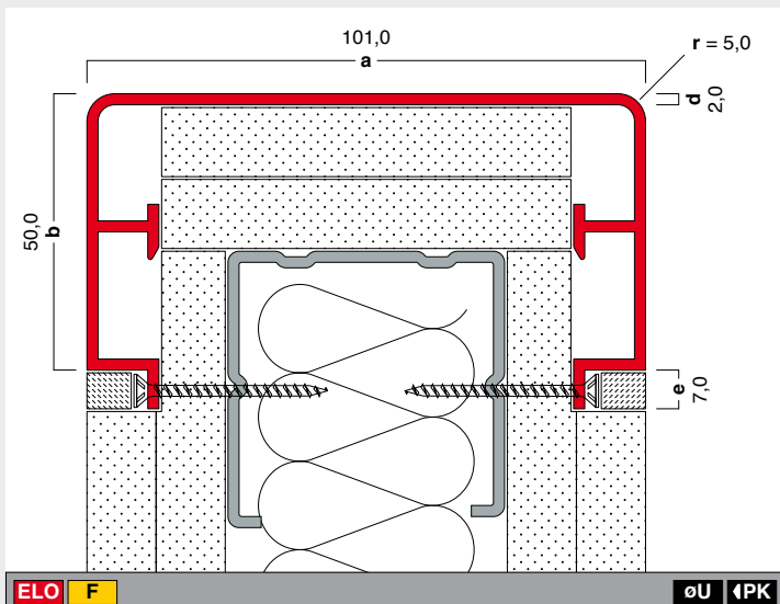
WA-ELO Aluminium-Wandabschluss im Trockenbau
