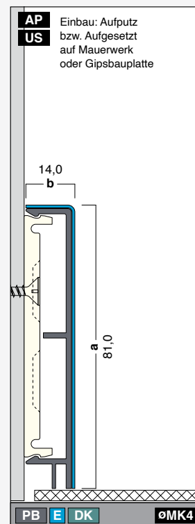
G81-14-DK-E Höhe: 81,0 mm Breite: 14,0 mm Länge: 2,0 / 2,5 / 3,0 m
