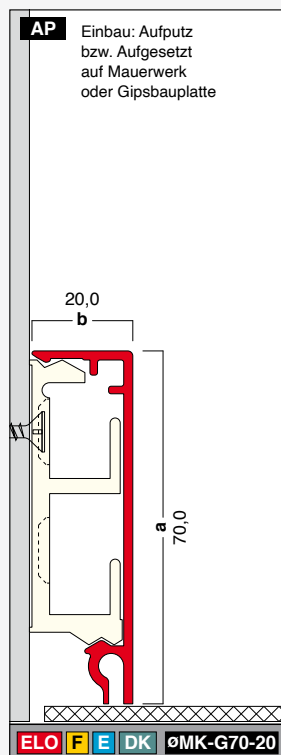
G70-20-DK Höhe: 70,0 mm Breite: 20,0 mm Länge: 4,0 m
