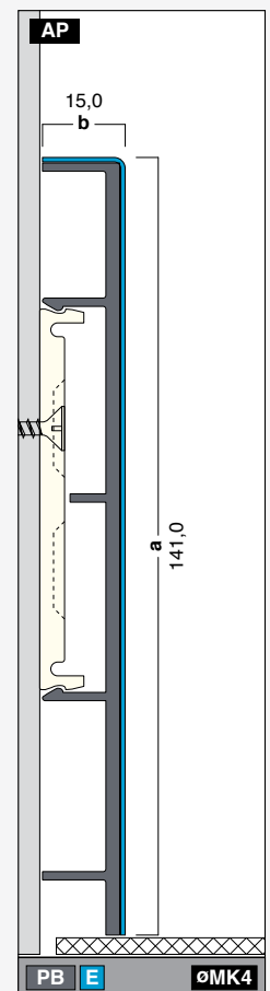
G141-15-E Höhe: 141,0 mm Breite: 15,0 mm Länge: 2,0/2,5/3,0 m
