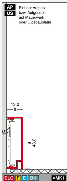
G43-13-DK Höhe: 43,0 mm Breite: 13,0 mm Länge: 4,0 m
