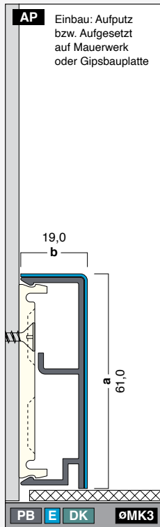
G61-19-DK-E Höhe: 61,0 mm Breite: 19,0 mm Länge: 2,0/2,5/3,0 m G60x18-E
