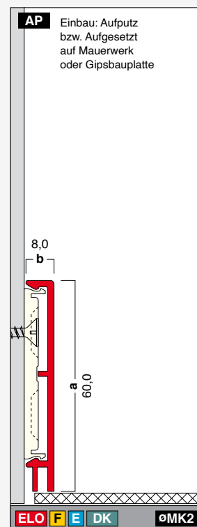
G60-8-DK Höhe: 60,0 mm Breite: 8,0 mm Länge: 4,0 m
