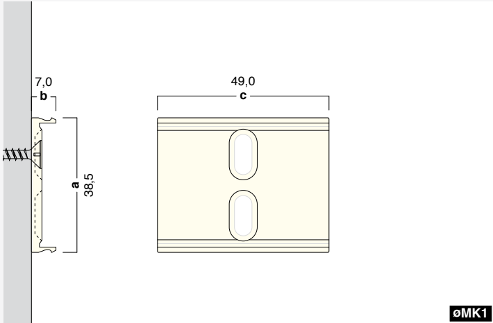
MK1 – 39-7-49 – Montageklipse 1 Serie G
