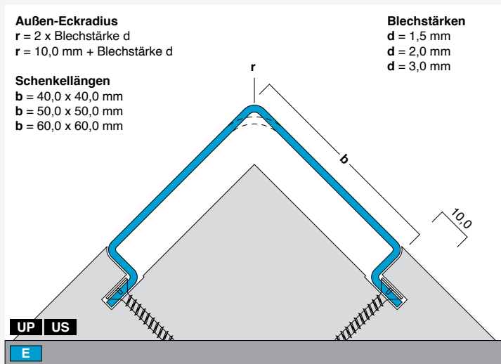
ES11-E Profillänge (Höhe): 2,0 / 2,5 / 3,0 m ES11/90°
