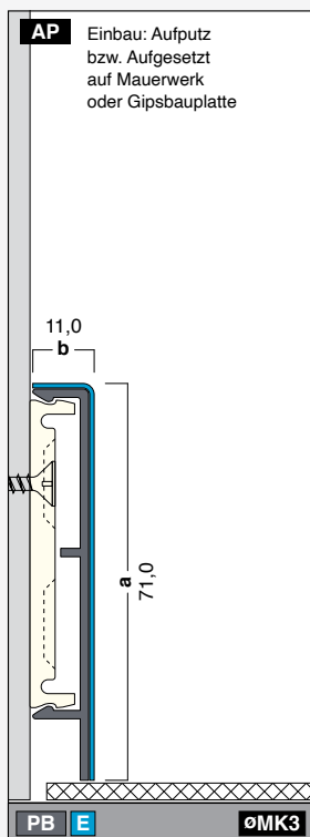
G71-11-E Höhe: 71,0 mm Breite: 11,0 mm Länge: 2,0 / 2,5 / 3,0 m
