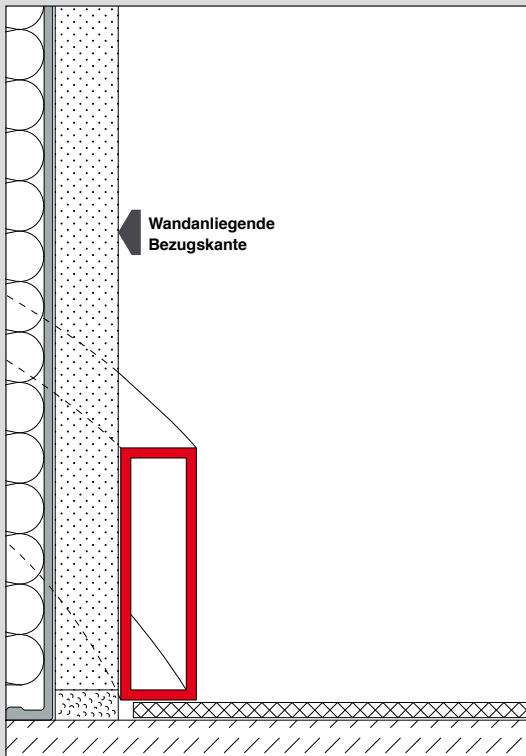
R-Profil Konvex R50-15-2 „Konvex“ gebogen
