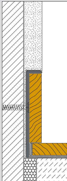
Unterputz-Einbau mit Holz- / Laminatboden 10,0 mm
