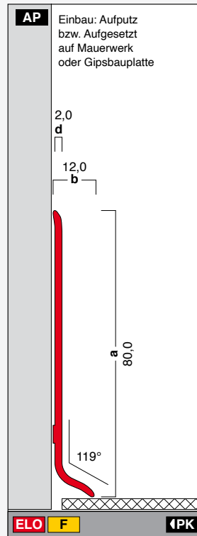
XL80-12 Höhe: 80,0 mm Breite: 12,0 mm Länge: 4,0 m XL8012
