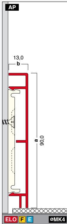
G90-13-DK Höhe: 90,0 mm Breite: 13,0 mm Länge: 4,0 m
