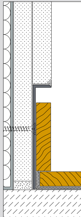
Unterschnittener Einbau mit Holz- / Laminatboden und einer Schattenfuge
