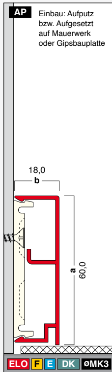
G60-18-DK Höhe: 60,0 mm Breite: 18,0 mm Länge: 4,0 m
