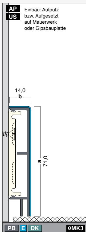
G71-14-DK-E Höhe: 71,0 mm Breite: 14,0 mm Länge: 2,0 / 2,5 / 3,0 m
