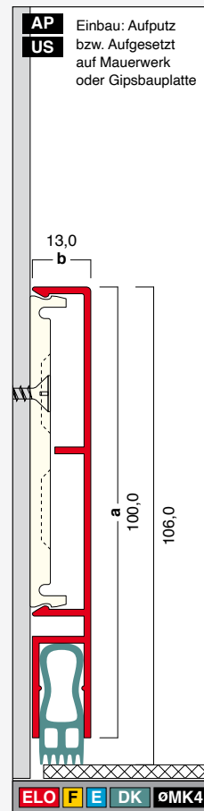
G106-13-DK Höhe: 106,0 mm Breite: 13,0 mm Länge: 4,0 m
