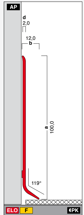
XL100-12 Höhe: 100,0 mm Breite: 12,0 mm Länge: 4,0 m XL10012
