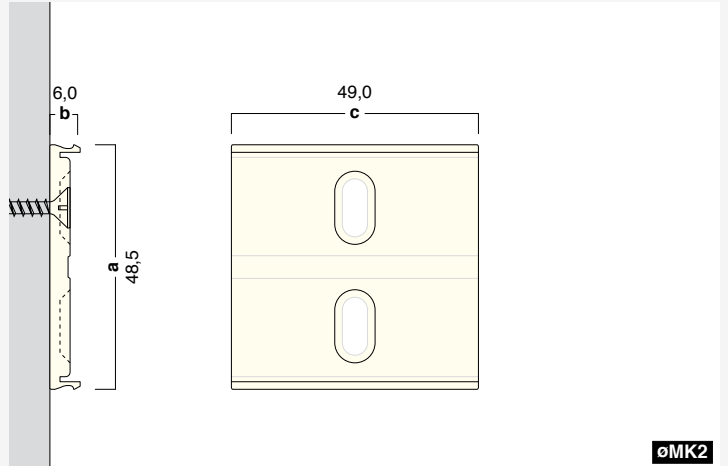
MK2 – 49-6-49 – Montageklipse 2 Serie G
