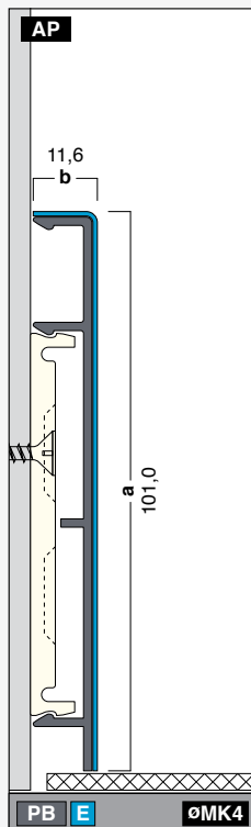
G101-12-E Höhe: 101,0 mm Breite: 11,6 mm Länge: 2,0/2,5/3,0 m G2-E
