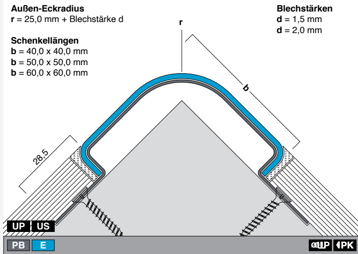
ES9-OP-E ES9-UP-PB Profillänge (Höhe): 2,0 / 2,5 / 3,0 m ES9/90°
