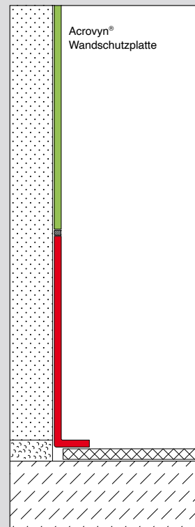
Profil L60-10-2-ELO mit einer Acrovyn® Wand- schutzplatte
