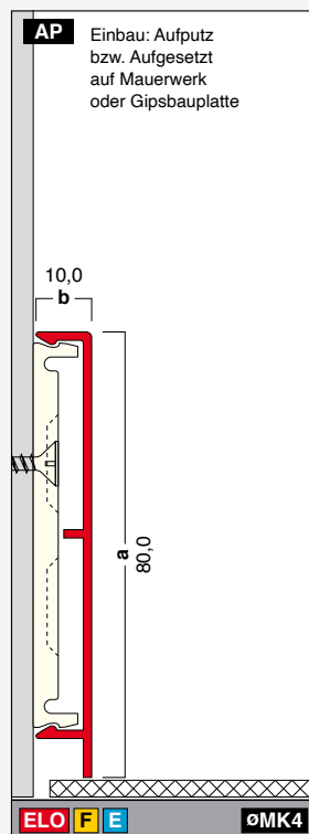
G80-10 Höhe: 80,0 mm Breite: 10,0 mm Länge: 4,0 m
