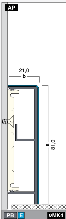
G81-21-E Höhe: 81,0 mm Breite: 21,0 mm Länge: 2,0/2,5/3,0 m G80x20-E
