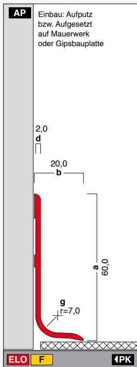
XL60-20 Höhe: 60,0 mm Breite: 20,0 mm Länge: 4,0 m XL6020
