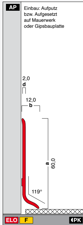
XL60-12 Höhe: 60,0 mm Breite: 12,0 mm Länge: 4,0 m XL6012
