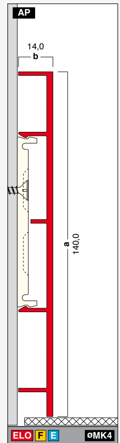
G140-14 Höhe: 140,0 mm Breite: 14,0 mm Länge: 3,0 m
