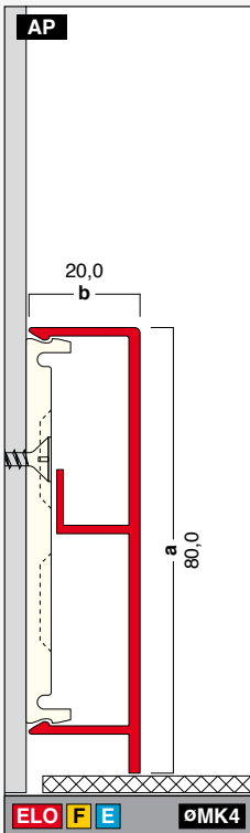
G80-20 Höhe: 80,0 mm Breite: 20,0 mm Länge: 4,0 m
