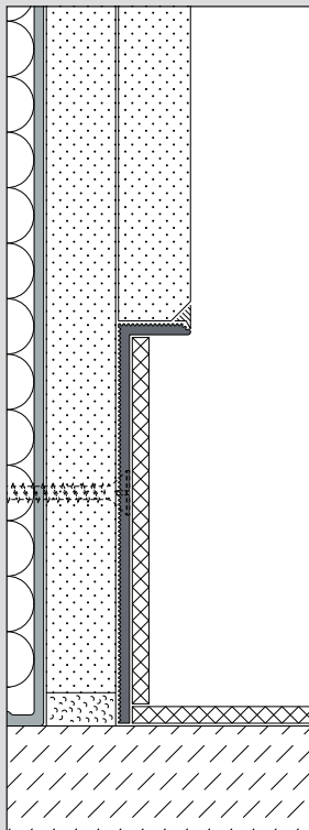
Unterschnittener-Einbau mit PVC-Bodenbelag 3,0 mm
