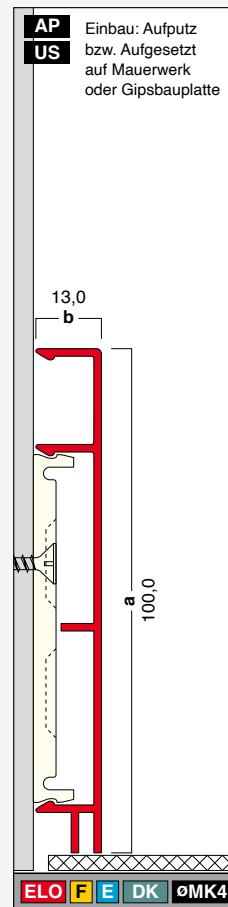
G100-13-DK Höhe: 100,0 mm Breite: 13,0 mm Länge: 4,0 m
