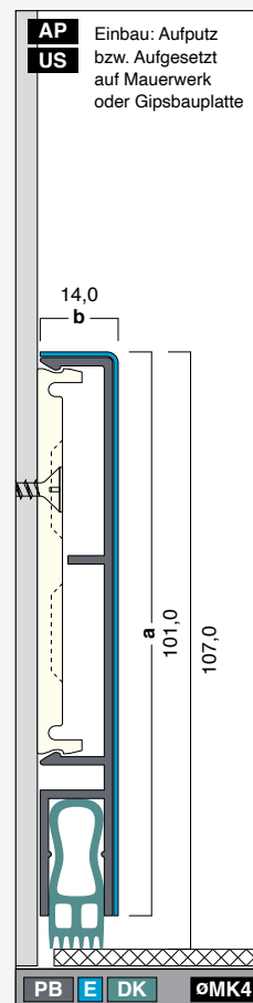
G107-14-DK-E Höhe: 107,0 mm Breite: 14,0 mm Länge: 2,0/2,5/3,0 m G11
