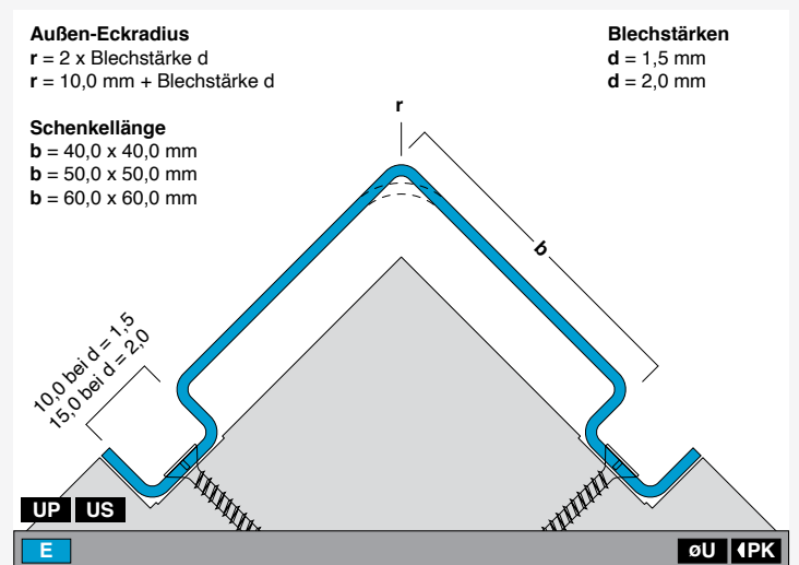
ES21-E Profillänge (Höhe): 2,0 / 2,5 / 3,0 m ES21/90°
