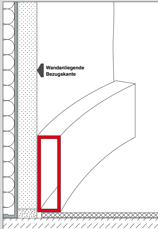
R-Profil Konkav R50-15-2 „Konkav“ gebogen
