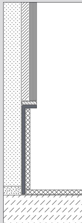
Profil L60-10-2-PB mit Wand-Fliesenbelag und Bodeneinlage
