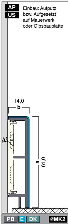
G61-14-DK-E Höhe: 61,0 mm Breite: 14,0 mm Länge: 2,0/2,5/3,0 m G6-E
