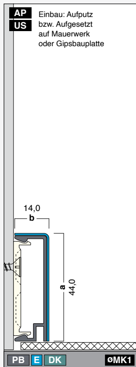
G44-14-DK-E Höhe: 44,0 mm Breite: 14,0 mm Länge: 2,0 / 2,5 / 3,0 m
