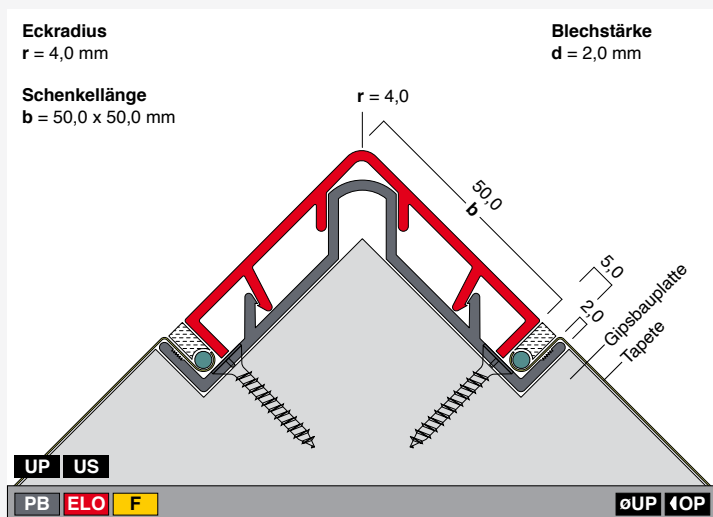
ES18-OP Profillänge (Höhe): 3,0 m
