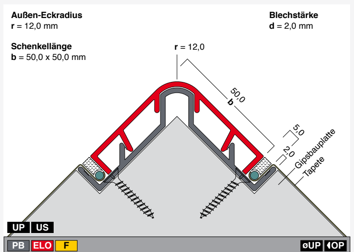
ES15-OP Profillänge (Höhe): 3,0 m
