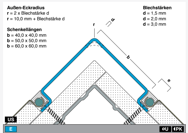
ES11-E Profillänge (Höhe): 2,0 / 2,5 / 3,0 m ES11/90°
