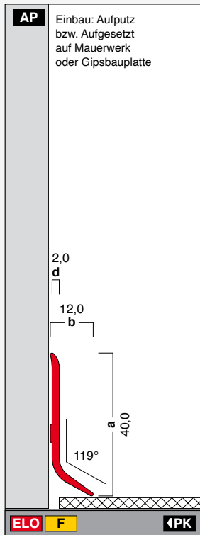
XL40-12 Höhe: 40,0 mm Breite: 12,0 mm Länge: 4,0 m XL4012
