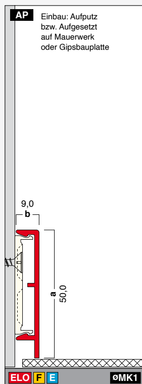
G50-9 Höhe: 50,0 mm Breite: 9,0 mm Länge: 4,0 m
