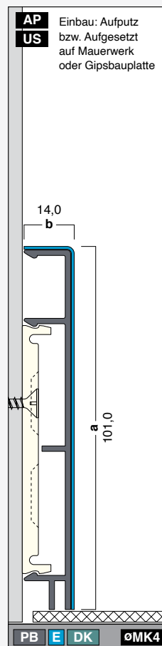
G101-14-DK-E Höhe: 101,0 mm Breite: 14,0 mm Länge: 2,0/2,5/3,0 m G10
