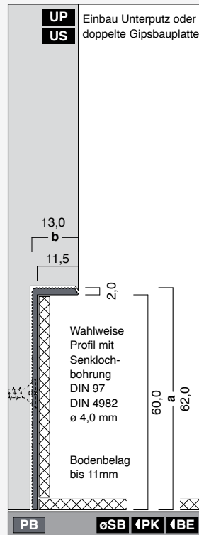
B62-13-BE11-RF-PB Höhe: 62,0 mm Breite: 13,0 mm Länge: 4,0 m
