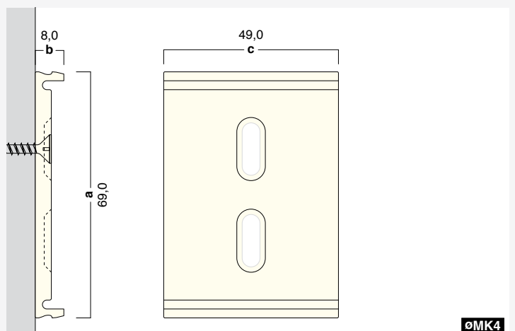
MK4 – 69-8-49 – Montageklipse 4 Serie G
