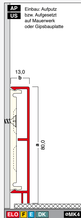
G80-13-DK Höhe: 80,0 mm Breite: 13,0 mm Länge: 4,0 m
