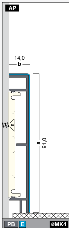
G91-14-DK-E Höhe: 91,0 mm Breite: 14,0 mm Länge: 2,0/2,5/3,0 m G4-E
