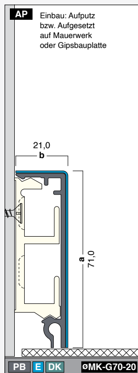
G71-21-DK-E Höhe: 71,0 mm Breite: 21,0 mm Länge: 2,0 / 2,5 / 3,0 m
