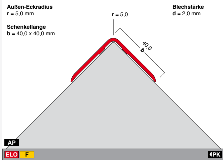
ESL1 Profillänge (Höhe): 3,0 m
