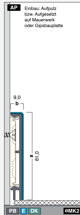
G61-9-DK-E Höhe: 61,0 mm Breite: 9,0 mm Länge: 2,0 / 2,5 / 3,0 m
