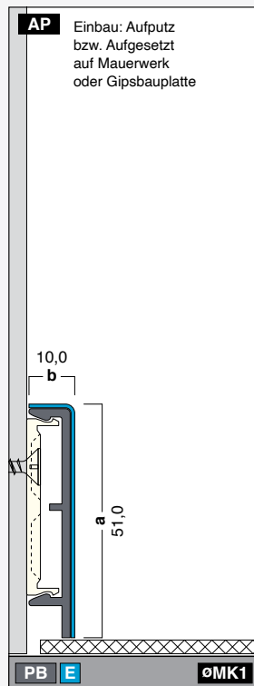
G51-10-E Höhe: 51,0 mm Breite: 10,0 mm Länge: 2,0 / 2,5 / 3,0 m
