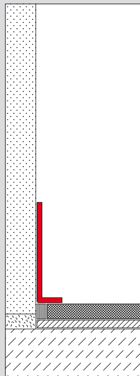
Profil L40-10-2-ELO als Dekorleiste auf Fliesenbelag
