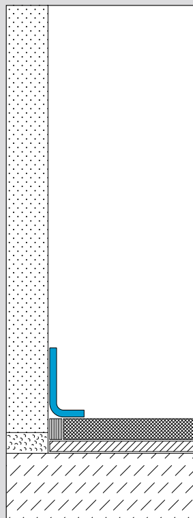
Profil L20-10-2-R2-E als Dekorleiste auf Fliesenbelag
