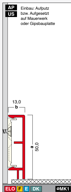
G50-13-DK Höhe: 50,0 mm Breite: 13,0 mm Länge: 4,0 m
