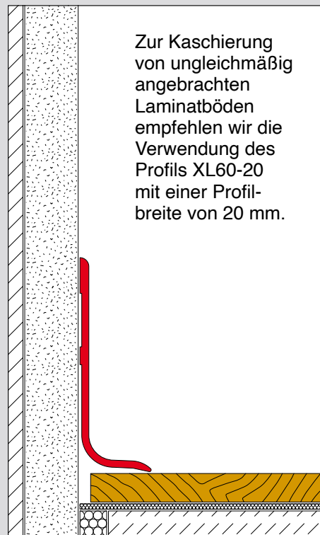
Aufputzprofil XL60-20-ELO mit Laminat- / Holzbodenbelag von 8 mm
