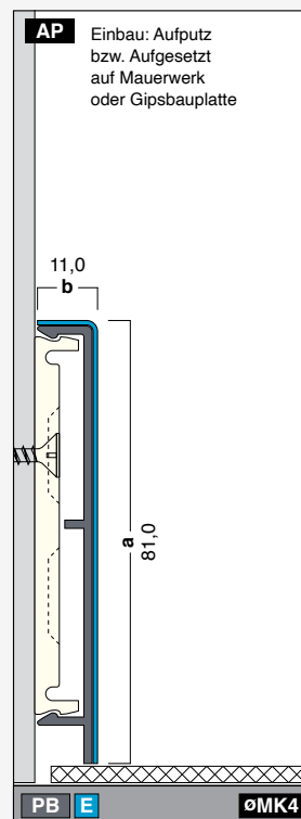
G81-11-E Höhe: 81,0 mm Breite: 11,0 mm Länge: 2,0 / 2,5 / 3,0 m
