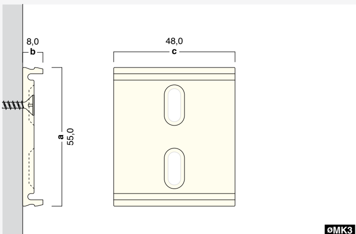
MK3 – 55-8-48 – Montageklipse 3 Serie G
