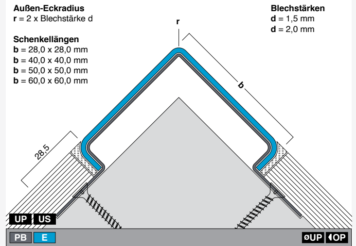
ES10-OP-E ES10-UP-PB Profillänge (Höhe): 2,0 / 2,5 / 3,0 m ES10/90°
