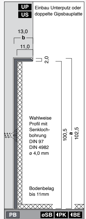
B103-13-BE11-RF-PB Höhe: 102,5 mm Breite: 13,0 mm Länge: 4,0 m
