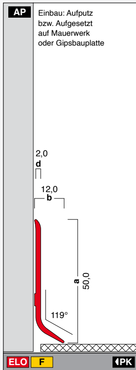
XL50-12 Höhe: 50,0 mm Breite: 12,0 mm Länge: 4,0 m XL5012
