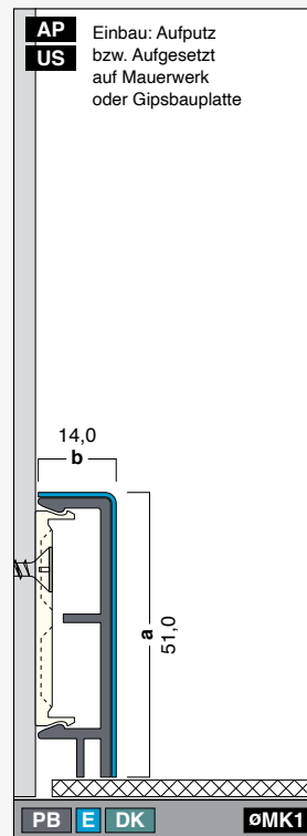
G51-14-DK-E Höhe: 51,0 mm Breite: 14,0 mm Länge: 2,0 / 2,5 / 3,0 m
