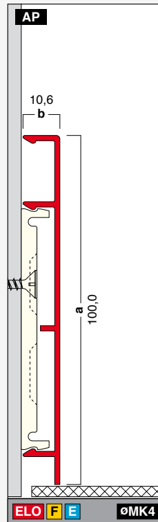
G100-11 Höhe: 100,0 mm Breite: 10,6 mm Länge: 4,0 m
