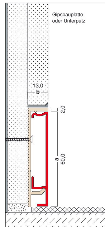
X60/F1 60,0 x 13,0 mm
