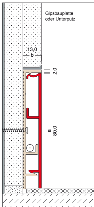
X80/F1 80,0 x 13,0 mm
