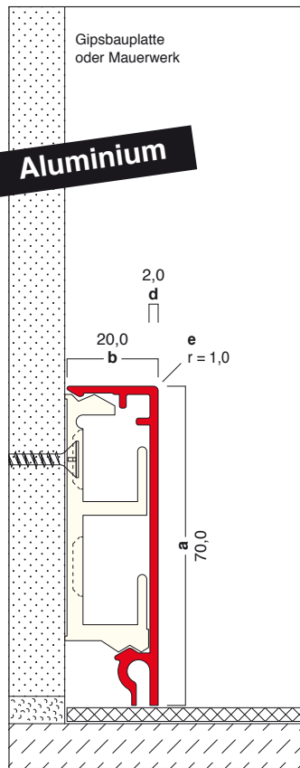
K1 70,0 x 20,0 mm
