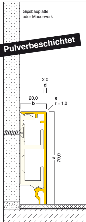
K1-F 70,0 x 20,0 mm
