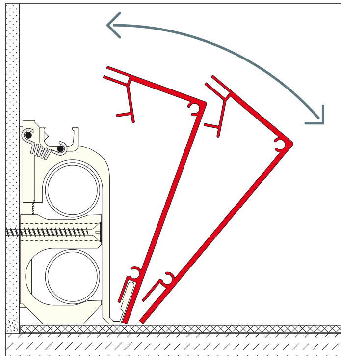
Die Profile K1, K2 und K3 sind in Aluminium, mit einer Edelstahlaufladdoppelung oder Pulverbeschichtet lieferbar!
